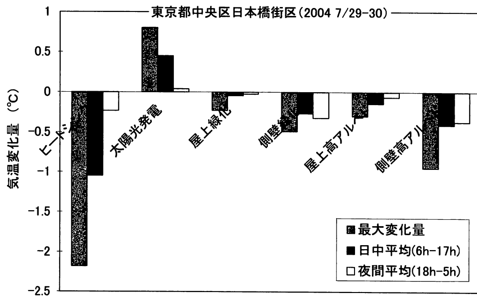
図8 各種ケース導入時と未導入時の地上気温差 (各ケースー標準ケース) の最大量・日中平均・夜間平均. 正値が気温上昇, 負値が気温低下を表す.
